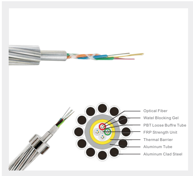
▲ OPGW cable
