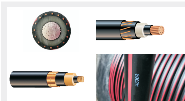
▲ MV URD cable //
